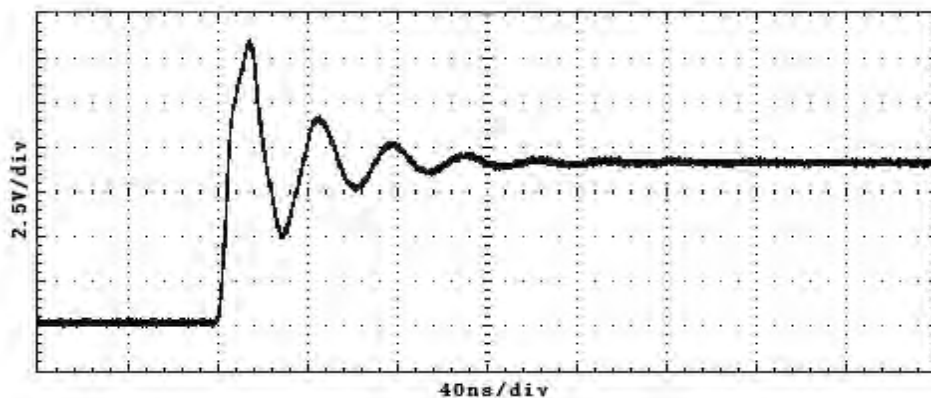
添加输入延长线(CK-301)的波形
