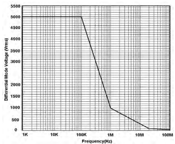
图 4: VP5210A/VP5215A 最大差模电压 VS 频率
