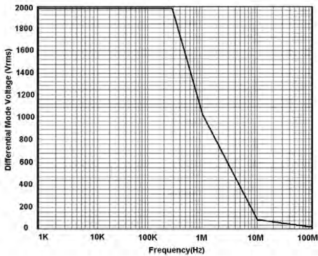
图 3: VP5208A 最大差模电压 VS 频率
