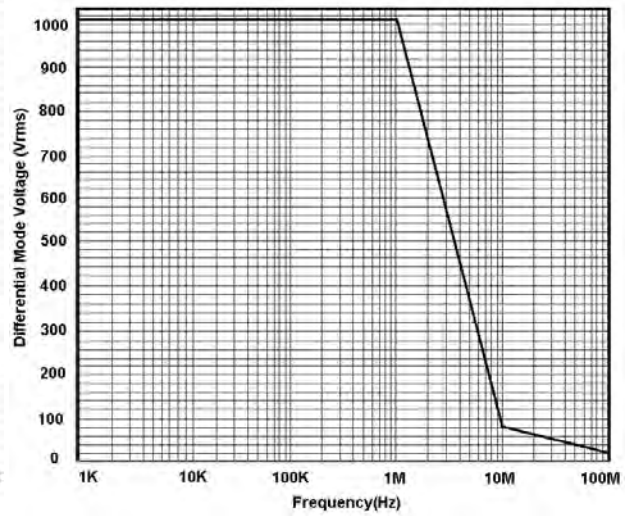
图 2: VP5200A/VP5205 (A/B) 最大差模电压 VS 频率
