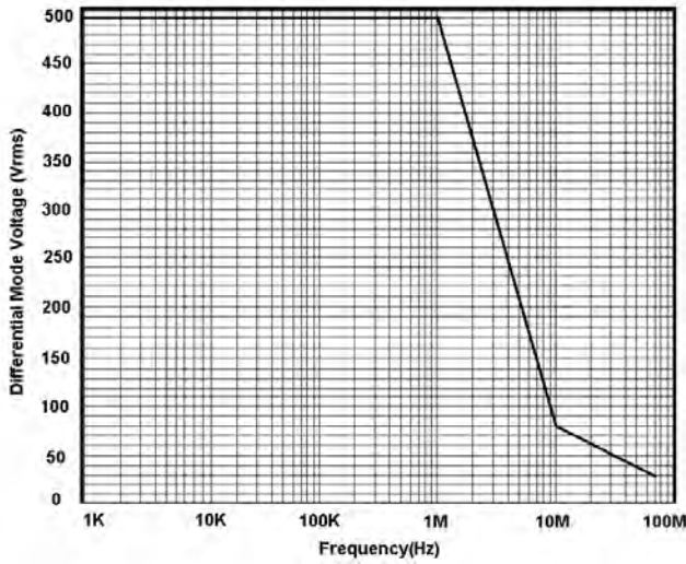
图 1: VP5065A 最大差模电压 VS 频率
